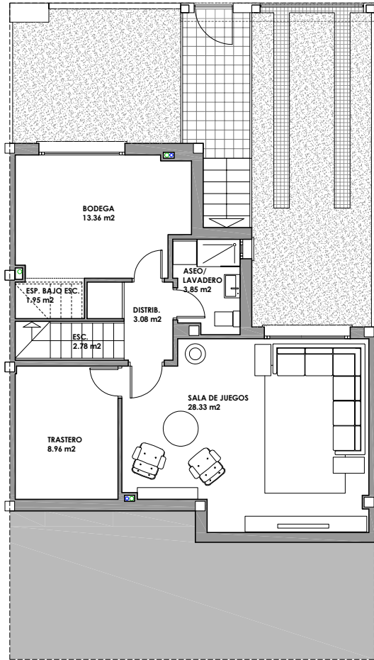
PLANTA SOTANO
