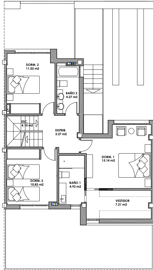
PLANTA PRIMERA
